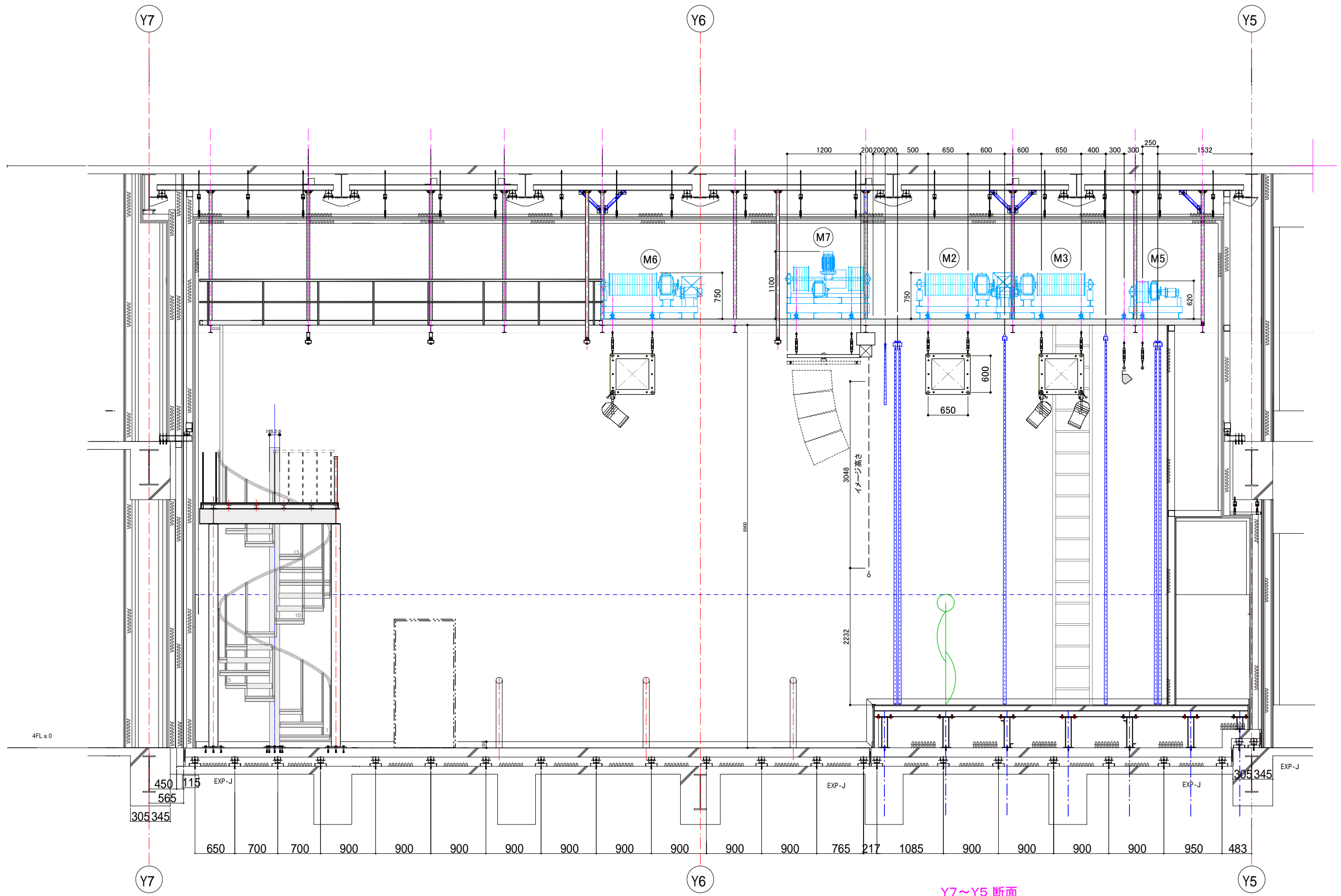
Y7~Y5 断面
